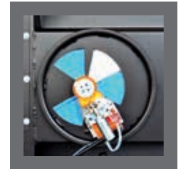
Verbrennungsluftdosierer geschlossen
