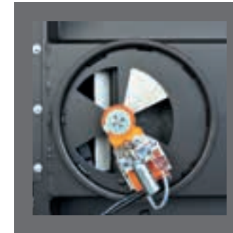
Verbrennungsluftdosierer offen
